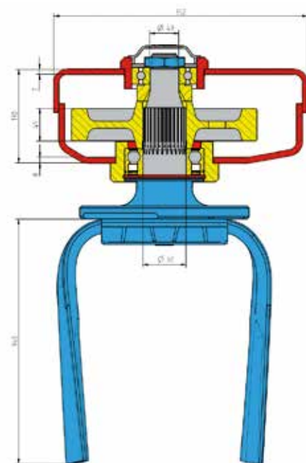
Vana ze silnostěnné kvalitní oceli (všechny údaje v mm)
